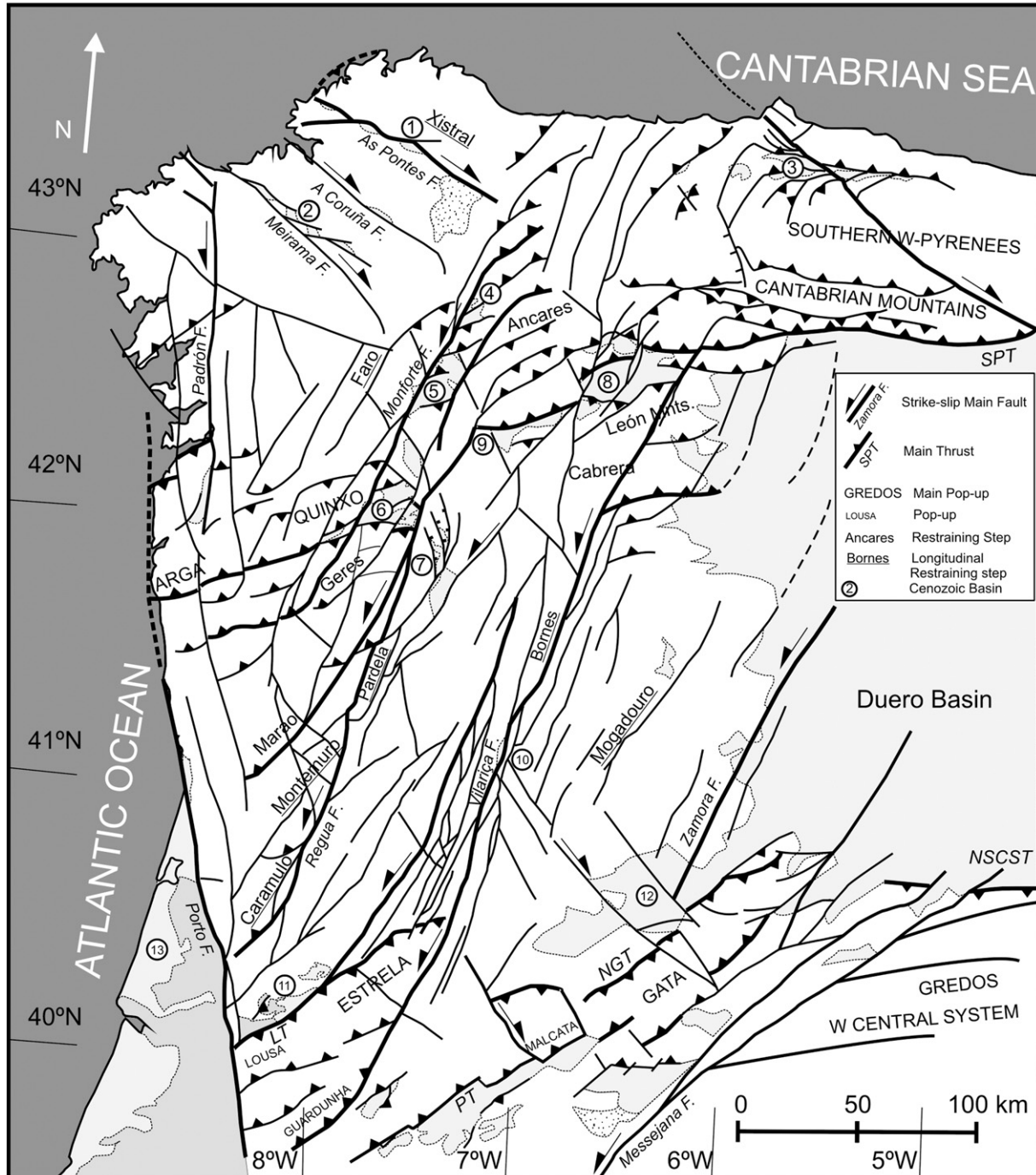
Fig. 7. Tectonic map of the distributed deformation of the Vilarica left lateral strike-slip fault system. Cenozoic Basins: 1) As Pontes. 2) Meirama. 3) Oviedo. 4) Sarria. 5) Monforte. 6) Xinzo. 7) Verín. 8) El Bierzo. 9) O Barco. 10) Vilarica. 11) Lousa. 12) Ciudad Rodrigo. 13) Lusitanian.
